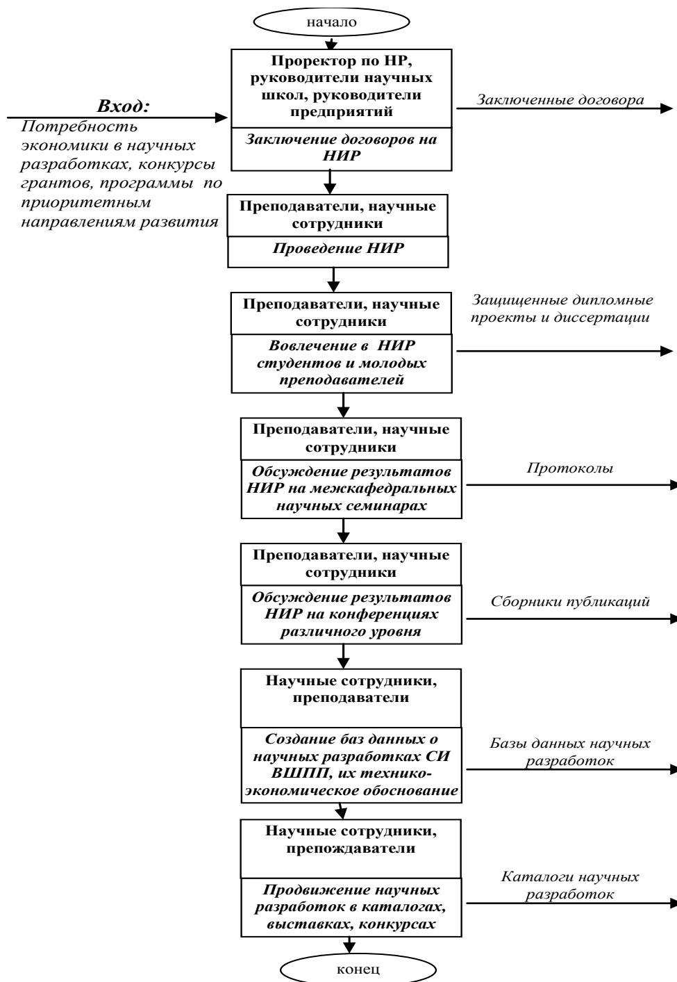
Рисунок 5. Алгоритм процесса "Научная деятельность"
